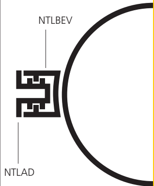
MAT SANS GORGE Ø 60 MM ET Ø 80 MM
