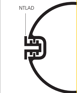
MAT AVEC GORGE Ø 60 MM ET Ø 90 MM
