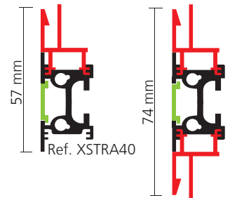
simple face double face
