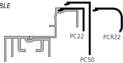
PROFILÉS LACUS ET DUO LACUS AVEC PARCLOSES DROITE PC22 OU PC50 OU PARCLOSES RONDE PCR22
