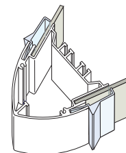
DÉTAIL DU PROFILÉ 87
