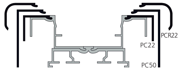
PROFILÉS LACUS ET DUO LACUS AVEC PARCLOSES DROITE PC22 OU PC50 OU PARCLOSES RONDE PCR22
