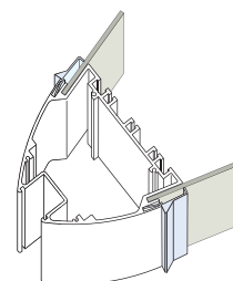
DÉTAIL DU PROFILÉ 157
